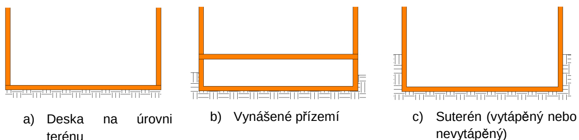
Obr 3.9: Typy přízemí
