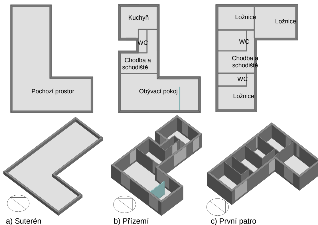
Fig. 4.8: Rozvržení podlaží
