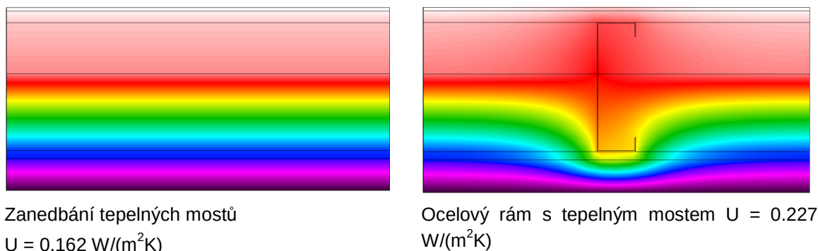
Obr. 3.11: Vliv tepelných mostů na hodnoty součinitele prostupu tepla pro lehký ocelový rám
