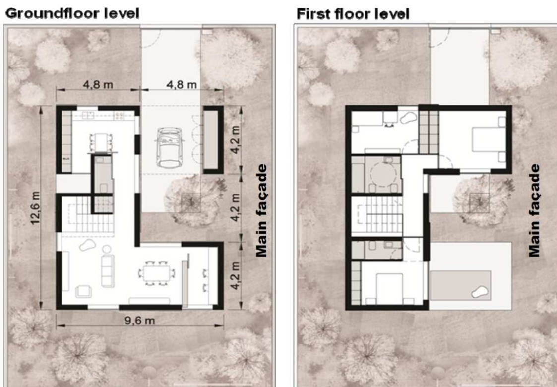
Obr. 4.2: Podlaží budovy
