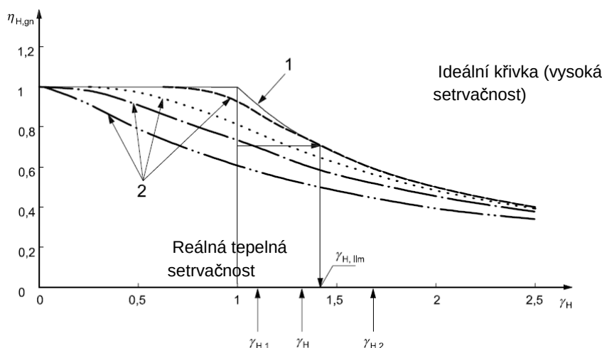
Obr. 3.10:Relevantní parametry pro stanovení části měsíce s potřebou energie pro chlazení a vytápění (ISO 13790)
