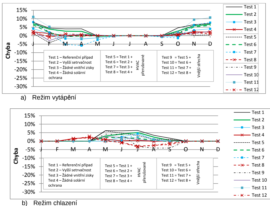
Obr. 3.13: Měsíční chyby algoritmu (měsíční kvazi-statická metoda)-referenční výsledky: Energy Plus (pokročilá dynamická metoda)
