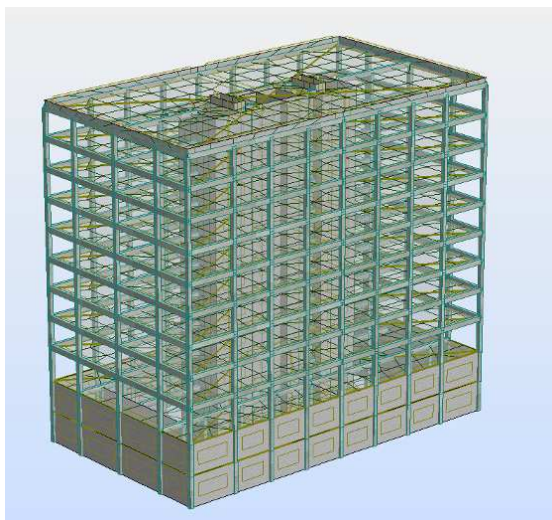
Obrázek 29 : Betonové jádro (Řešení 1 & 2)
