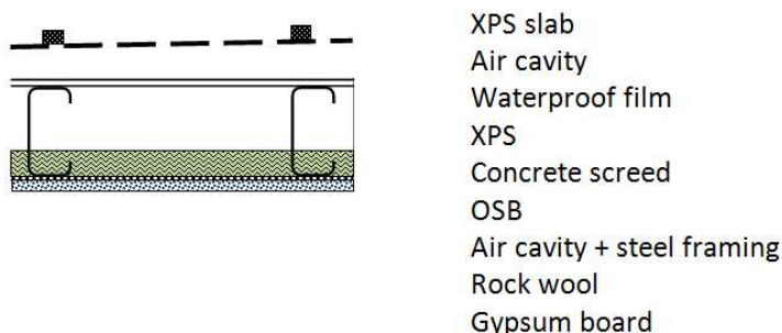
Obrázek 11 : typy skladby střechy, které jsou k dispozici v AMECO3
