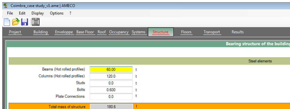
Obrázek 14 : Definování hmotnosti rozdílných ocelových konstrukčních prvků
